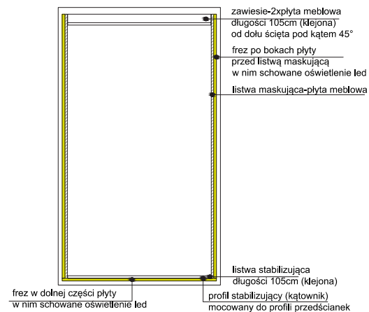
WIDOK_TYL PŁYTY
