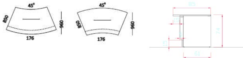
PRZEKRÓJ LADY NISKIEJ
