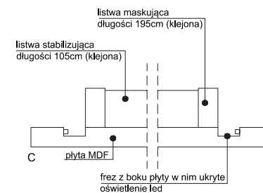
DETAL C I D PRZEKRÓJ POZIOMY SKALA 1:20
