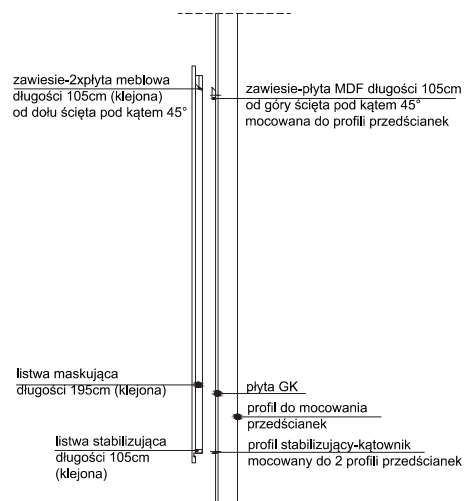
PRZEKRÓJ PIONOWY_SPOSÓB MONTAŻU PŁYTY
