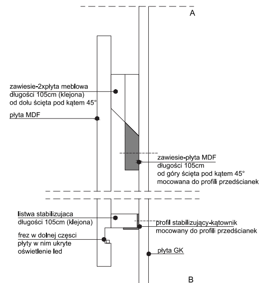
DETAL A I B PRZEKRÓJ PIONOWY SKALA 1:20
